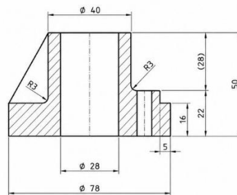
POTONGAN A-A
