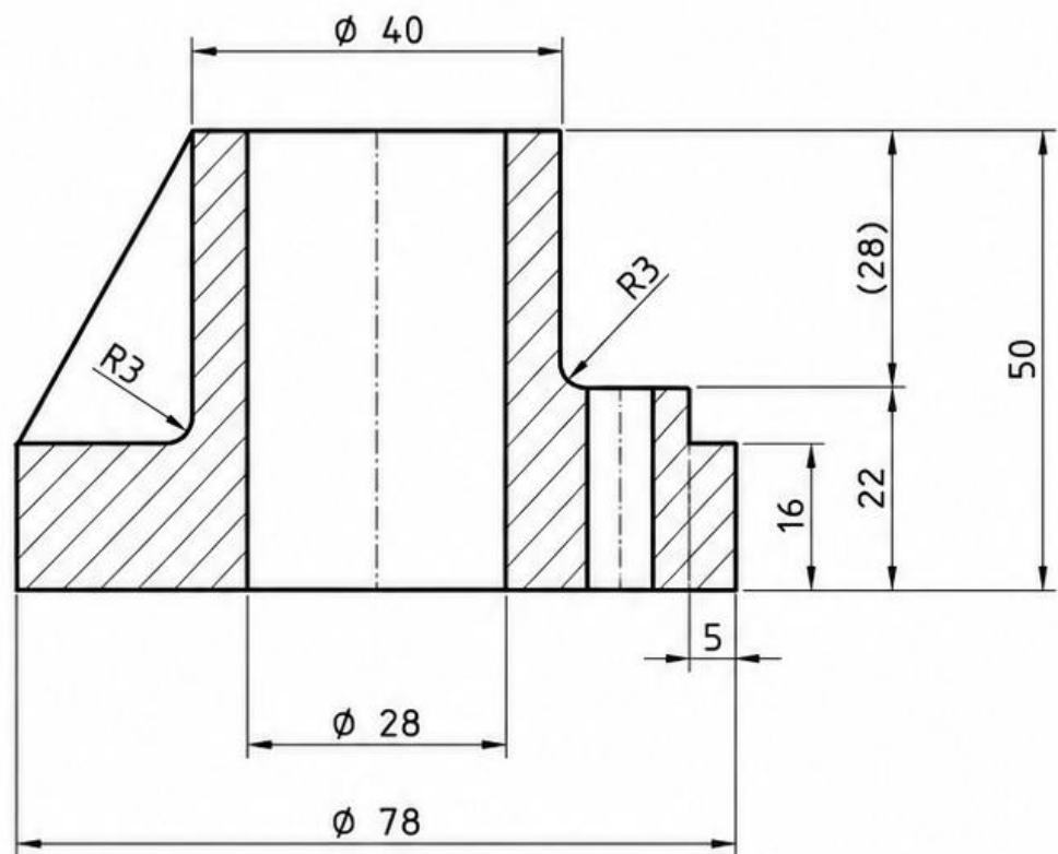
POTONGAN A-A
